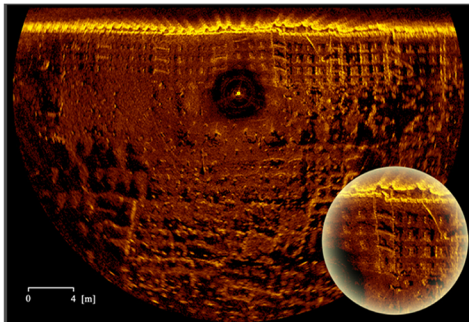
Inspekcja umocnień dna przy nabrzeżu portowym
