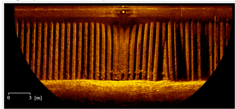
Inspekcja ścianki szczelnej
